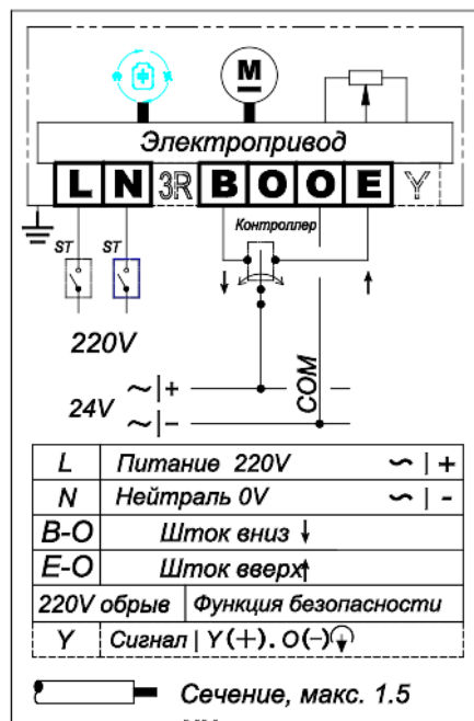
Импульсное управление, с аналоговым сигналом обратной связи
